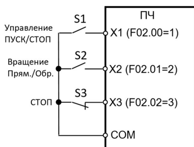
Трёхпроводное управление F00.03=3
