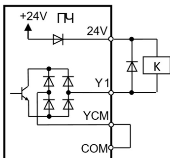
Логика NPN от внутреннего источника питания «24V».
