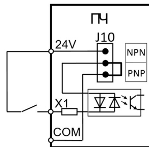
Логика PNP от внутреннего источника питания «+24V». Переключатель J10 в положении PNP.
