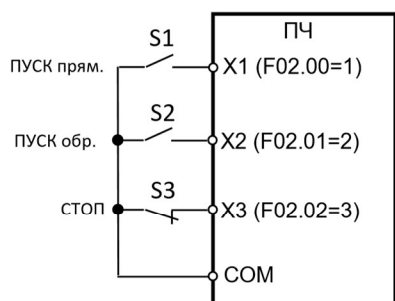
Трёхпроводное управление F00.03=2
