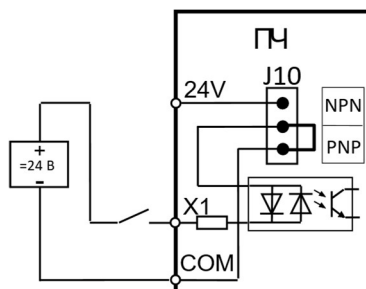
Логика PNP от внешнего источника питания 24 В. Переключатель J10 в положении PNP.
