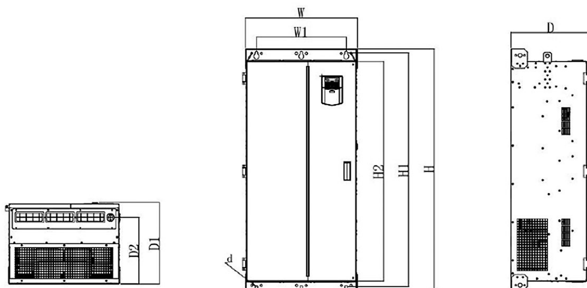
Рисунок 5 315...450 кВт (400Н...550Н)
