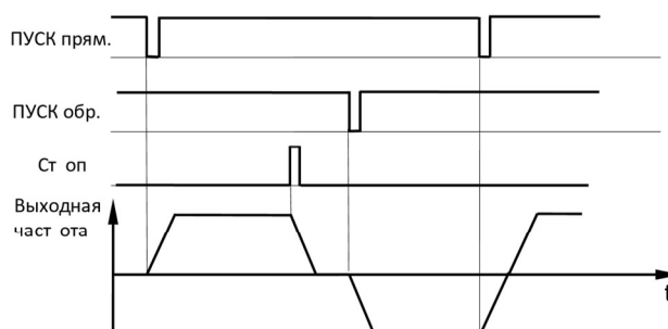
Трёхпроводное управление F00.03=2, F04.19=0
