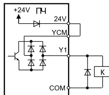
Логика PNP от внутреннего источника питания «24V».
