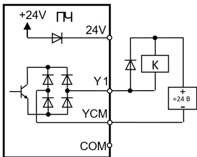
Логика NPN от внешнего источника питания 24V.
