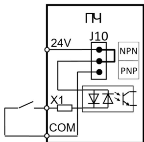
Логика NPN от внутреннего источника питания «+24V». Переключатель J10 в положении NPN.
