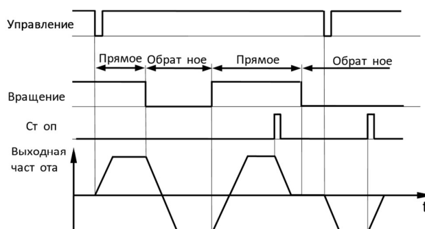
Трёхпроводное управление F00.03=3, F04.19=0
