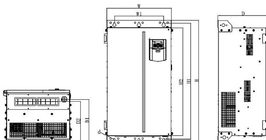
Рисунок 4 220 кВт (300H)
