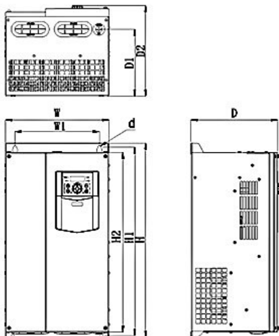
Рисунок 2 30...75 кВт (040H...100H)
