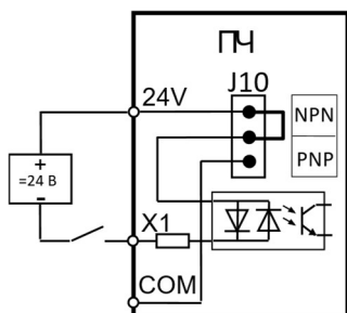
Логика NPN от внешнего источника питания 24 В. Переключатель J10 в положении NPN.
