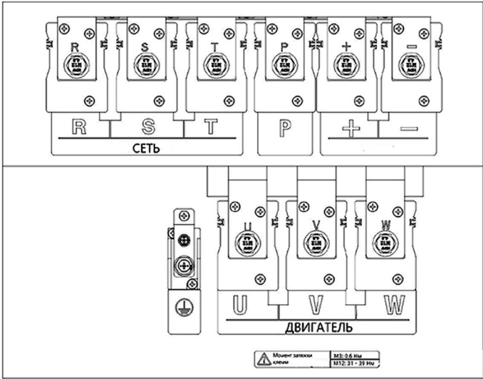
132, 160 кВт (175H...200H)
