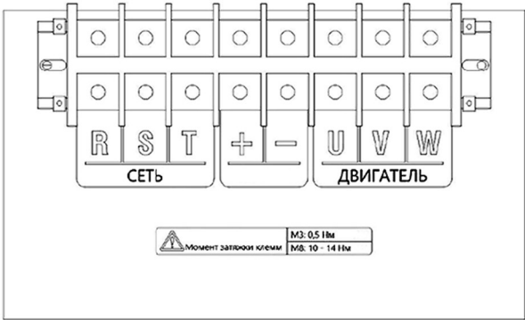
45...110 кВт (060H...150H)
