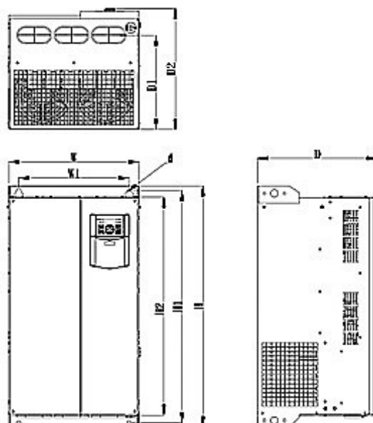
Рисунок 3 93...160 кВт (125H...200H)
