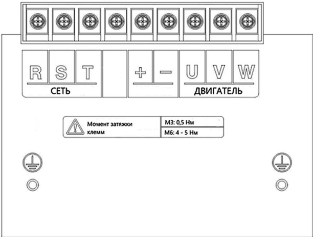
30, 37 кВт (040H, 050H)
