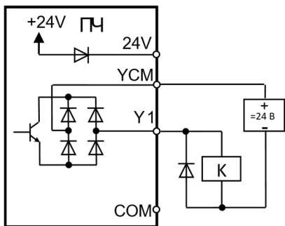
Логика PNP от внешнего источника питания 24V.
