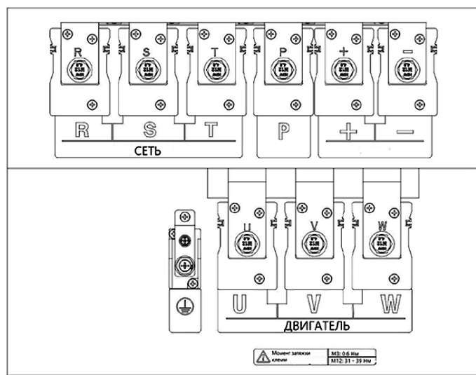
132, 160 кВт (175H...200H)
