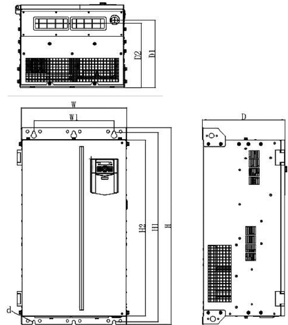
Рисунок 4 220 кВт (300H)
