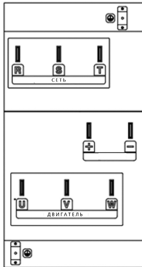
315...400 кВт (400H...500H)
