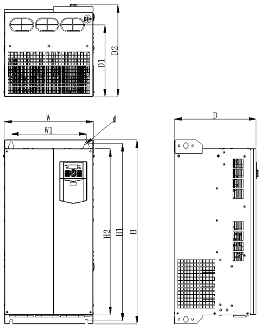
Рисунок 3 93...160 кВт (125H...200H)
