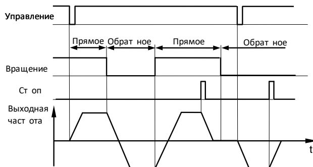
Трёхпроводное управление F00.03=3, F04.19=0
