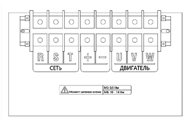
45...110 кВт (060H...150H)
