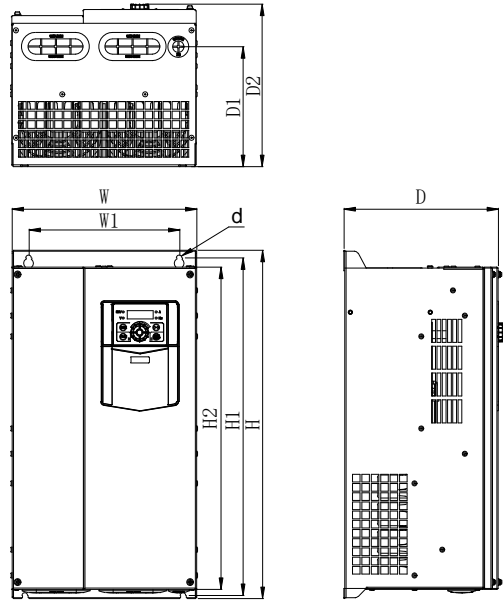
Рисунок 2 30...75 кВт (040H...100H)
