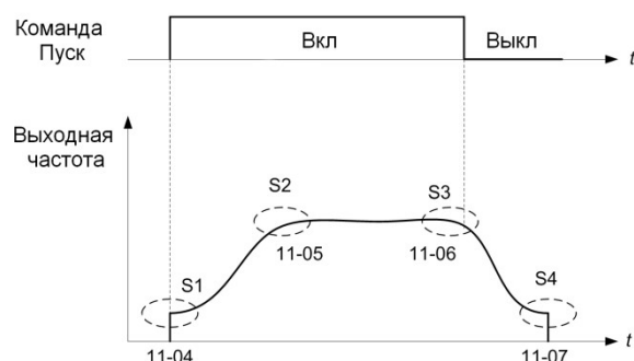
Рис. 4.3.85 S-кривые разгона / торможения
