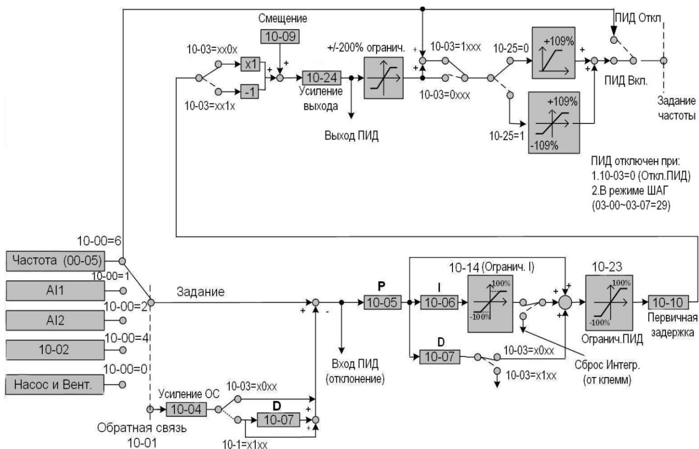
Рис. 4.3.81 Блок-схема ПИД-регулятора
