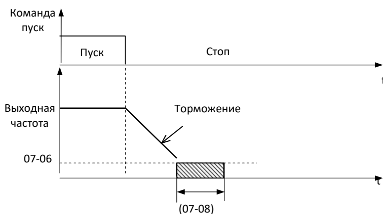
Рис.4.3.58 Плавный останов
