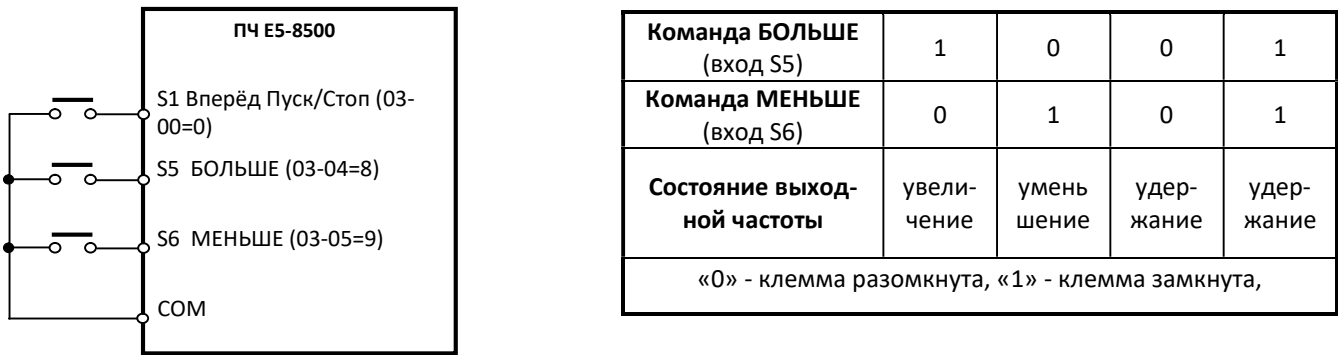
Рис.4.3.19 Пример управления в режиме БОЛЬШЕ/МЕНЬШЕ
