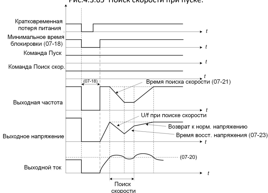
Рис. 4.3.66 Поиск скорости после кратковременной потери питания.
