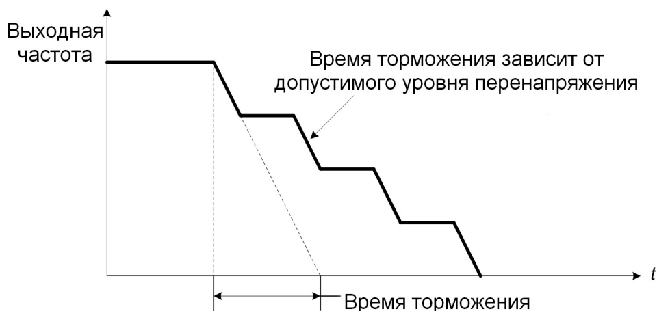
Рис. 4.3.69 Предотвращение срыва при торможении.
