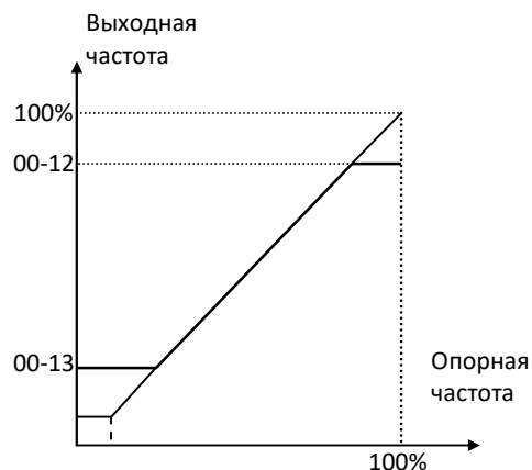
Рис. 4.3.6 Установка верхнего и нижнего пределов
