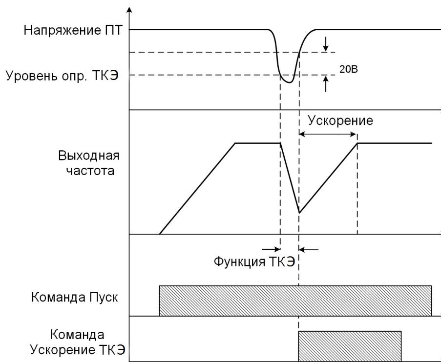
Рис. 4.3.95 Режим ТКЭ
