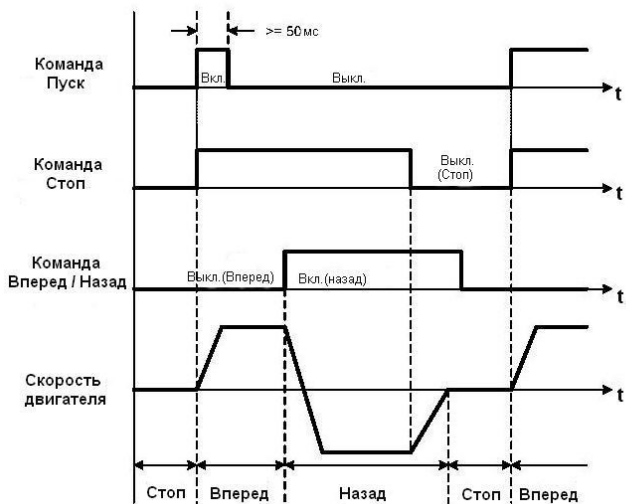
Рис.4.3.3. Алгоритм управления.
