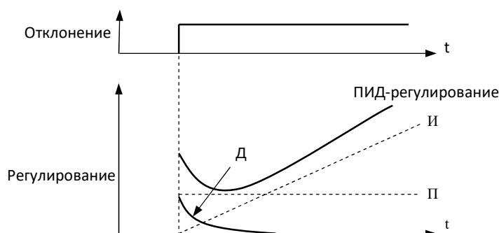
Рис. 4.3.79 ПИД-регулирование
