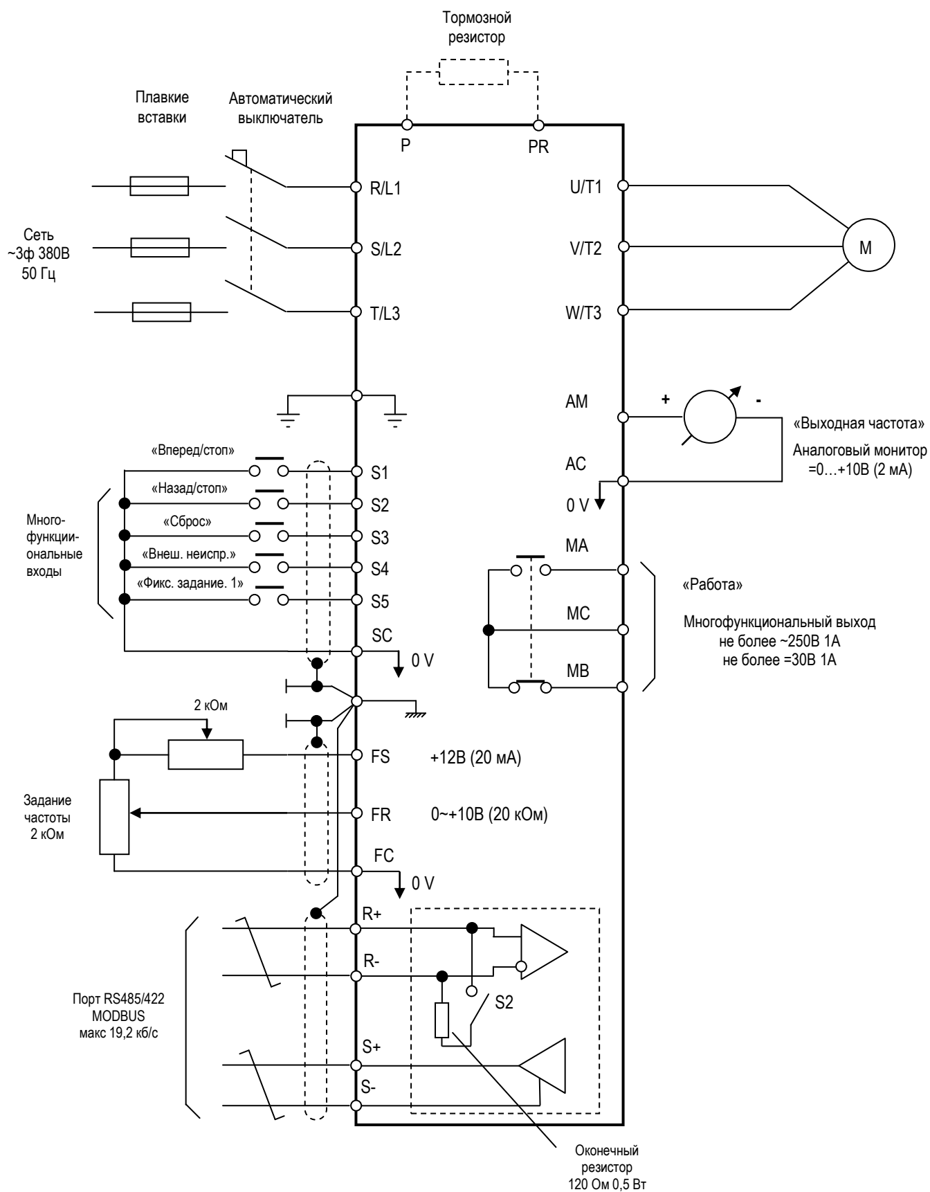
Схема подключения ЕЗ-8100В
