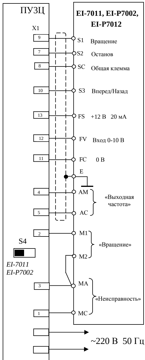
Схема подключения ПУЗЦ к EI-7011, EI-P7002
