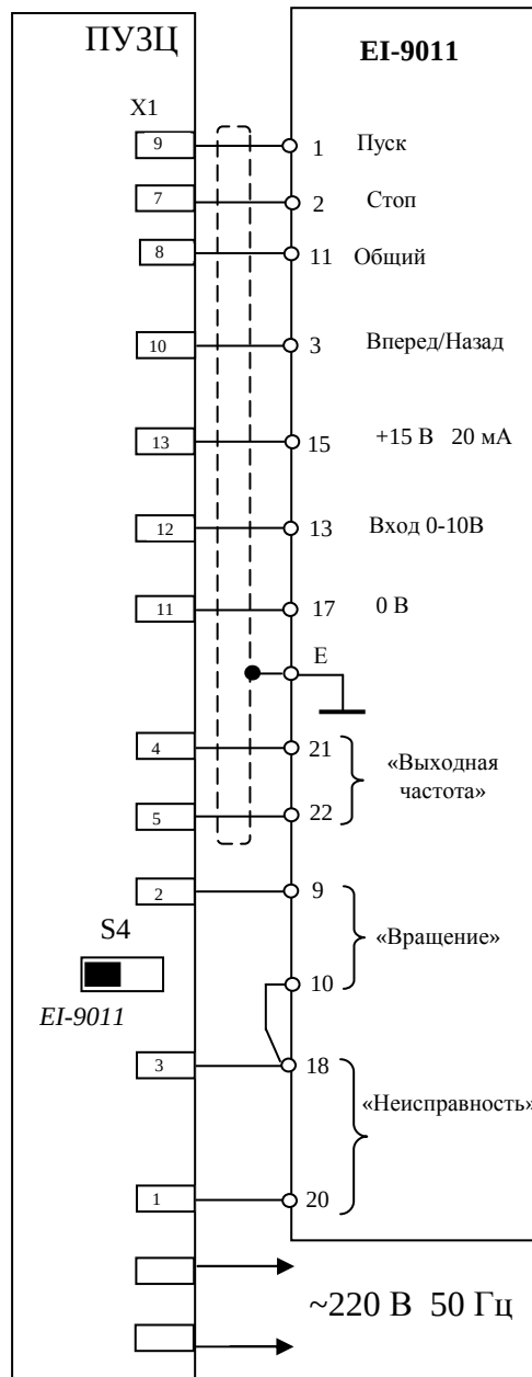
Схема подключения ПУЗЦ к EI-9011
