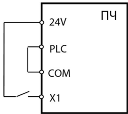
PNP (внутренний источник питания)
