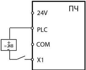
NPN (внешний источник питания)
