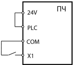
NPN (внутренний источник питания)
