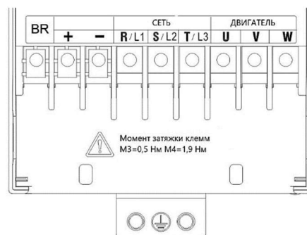
2,2...3,7 кВт (003Н, 005Н)
