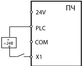
PNP (внешний источник питания)
